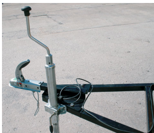
Fäste för dragkrok
